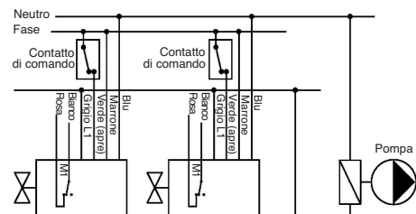
M1 MICROINTERRUTTORE SUPPLEMENTARE LIBERO IN APERTURA
