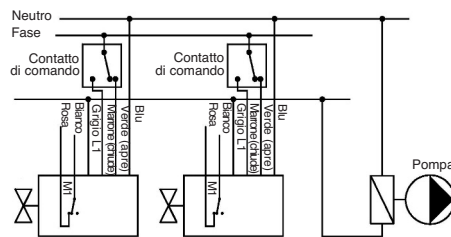
M1 MICROINTERRUTTORE SUPPLEMENTARE LIBERO IN APERTURA
